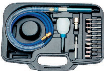
ATJ-3170 Микрошлифмашина в комплекте
