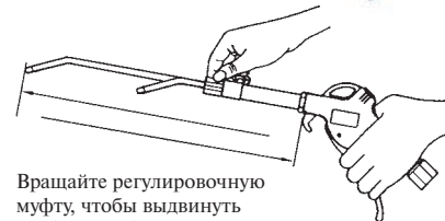
AA-5010 Пистолет обдувочный с регулируемым удлинителем
