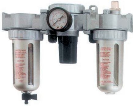
AA-2024 3/8" (1/2") фильтр, регулятор и лубрикатор
